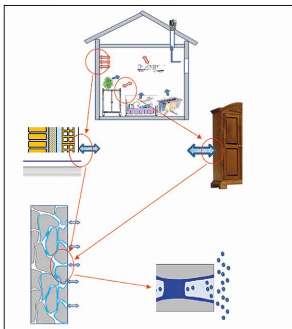
Figura 7.8. Esquema del fenómeno de moisture buffering desde el macro hasta el micro-nivel. Fuente: Gomez-Arriaran, Tesis Doctoral.
